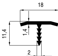
1138-180-00 T18 Geanodiseerd Anodisé
