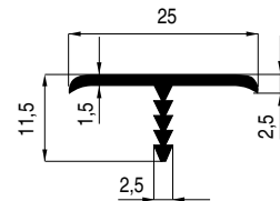
1138-250-00 T25 Geanodiseerd Anodisé
