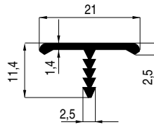
1138-215-00 T21 Geanodiseerd Anodisé
