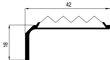
250-7631 Trapneus met rubber Nez d'escalier avec caoutchouc
